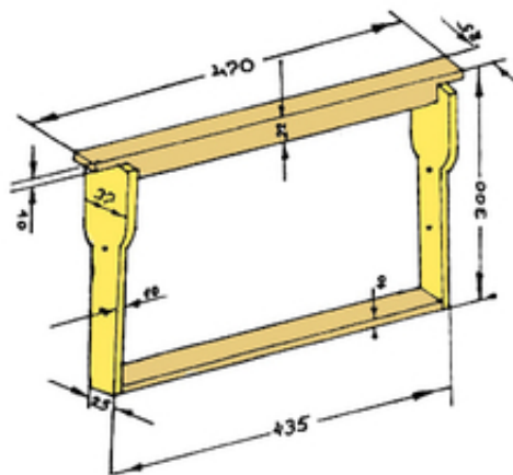
Гнездовая рамка Блатта в улье Дадана-Блатта
